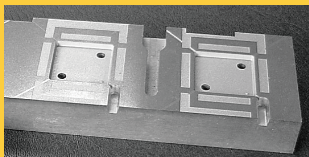
半導体モールド金型（セルテスX,N）
