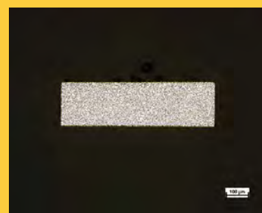
コネクター成形金型（セルテスX） ピン断面 0.8 x 0.2 mm
