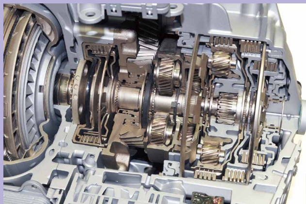
自動車・ロボット用駆動力伝達歯車（セルテス DT）
