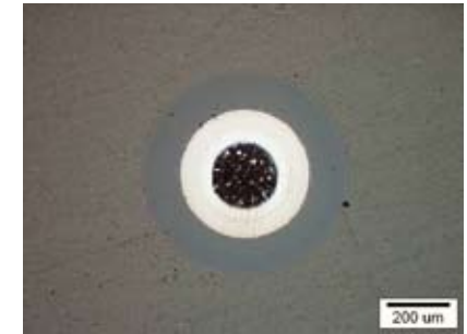
SKH51+下地層 0.6 μm/DLC 層 2.2 μm (エッチング)
